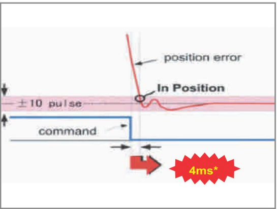
JSDAP系列高性能AC伺服马达拥有快速整定时间，反应快、响应高等特性。
